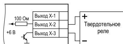
Рисунок 5.20 – Схема подключения нагрузки к ВУ типа «Т»
