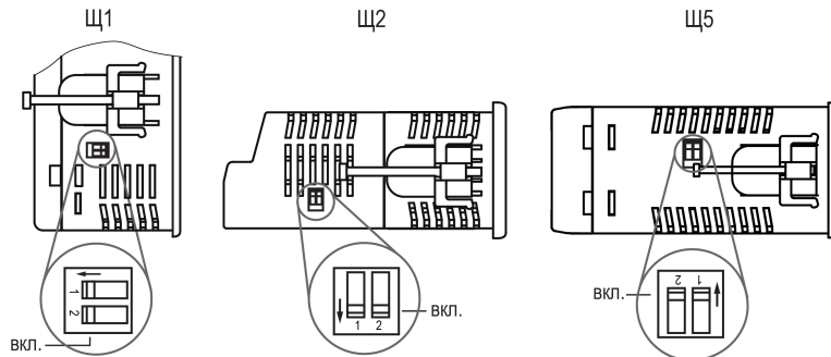
Рисунок 5.16 – Расположение DIP-переключателей
