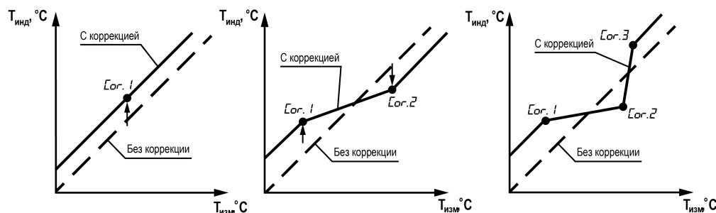
Рисунок 7.3 – Коррекция графика измерителя: T_{\text{изм}} — измеряемая температура, T_{\text{инд}} — температура, отображаемая на ЦИ
