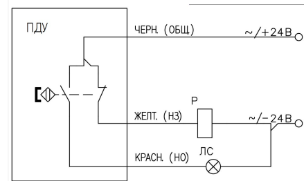
Рисунок 4.2 – Подключение датчика
