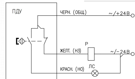
Рисунок 4.2 – Подключение датчика
