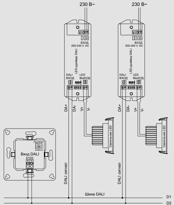
Схема установки 4
