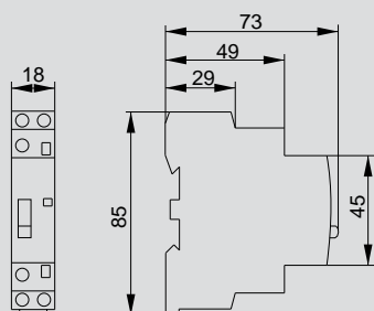
КМ20-11 MP AC, КМ20-20MP AC
