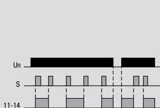
Функциональная диаграмма реле ORM 1 конт.
