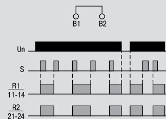
Функциональная диаграмма реле ORM-02. Режим управления 2
