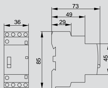
КМ20-22MP AC, КМ20-40MP AC, КМ25-22MP AC
