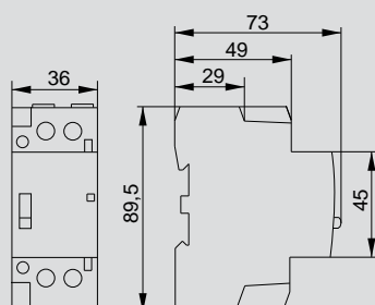
КМ40-11 MP AC, КМ40-20MP AC, КМ63-11 MP AC, КМ63-20MP AC
