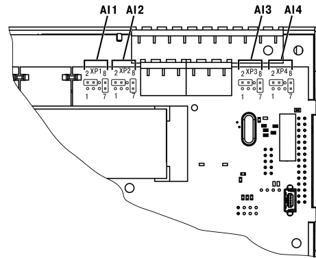
Рисунок 8.3 – Расположение входов
