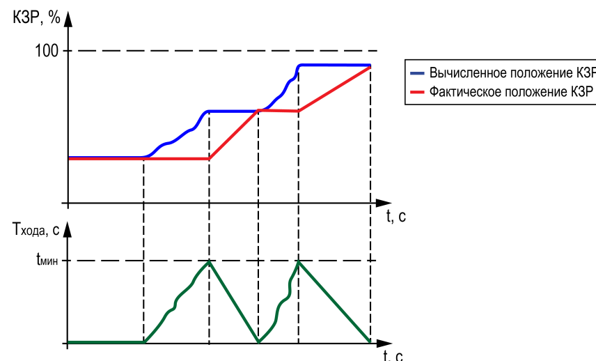
Рисунок 14.2 – Зависимость времени хода
