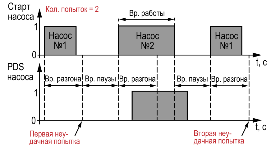
Рисунок 14.8 – Перезапуск насоса
