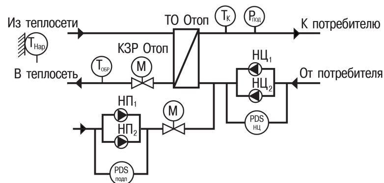
Рисунок 3.1 – Схема контура «Отопление»
