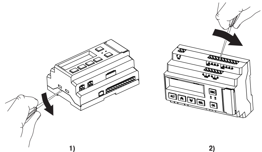
Рисунок 8.1 – Снятие верхней крышки
