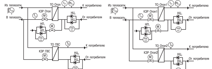
Рисунок 4 – Схема контура «Отопление + ГВС»
