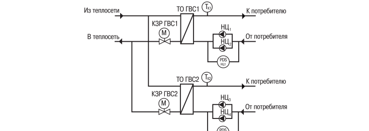
Рисунок 6 – Схема контура «ГВС + ГВС»
