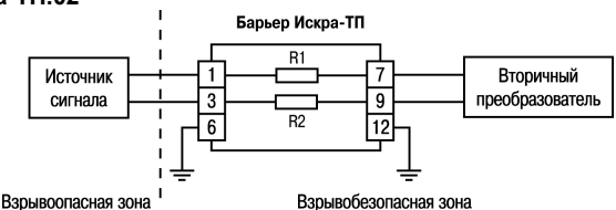
Рисунок 3.2 – Схема подключения барьера, R1=R2=110 \text{ Ом} \pm 5\%
