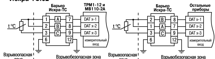
Рисунок 3.3 – Схема подключения барьера
